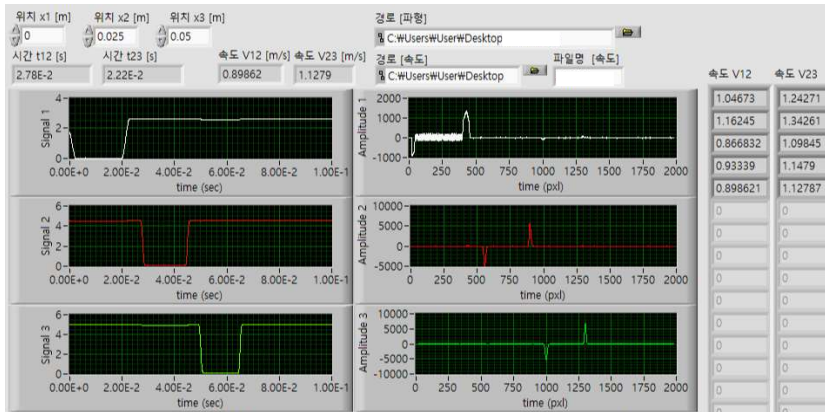
Software 화면
