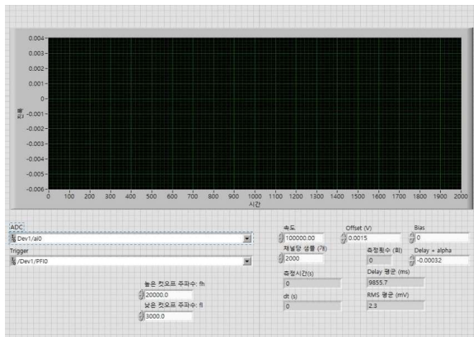
Software 화면
